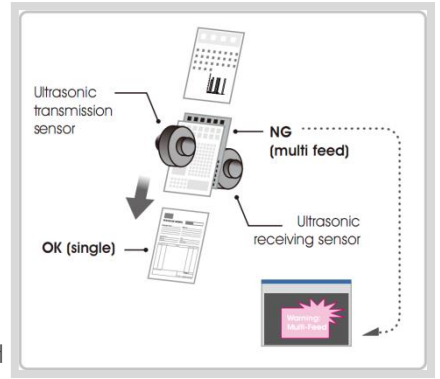
종이걸림을 최소화 하는 직선형 급지와 초음파센서
